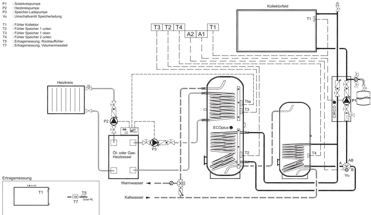
Abb. 4 Systemlösung für Warmwasserbereitung. Der Regler SUNGO SL sorgt für die solare Beladung eines bivalenten Solarspeichers und des vorgeschalteten Monovalentspeichers.
