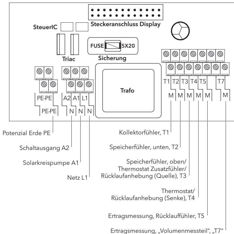
Abb. 2 Reglerplatine SUNGO SL mit Klemmenbelegung für elektrischen Anschluss
