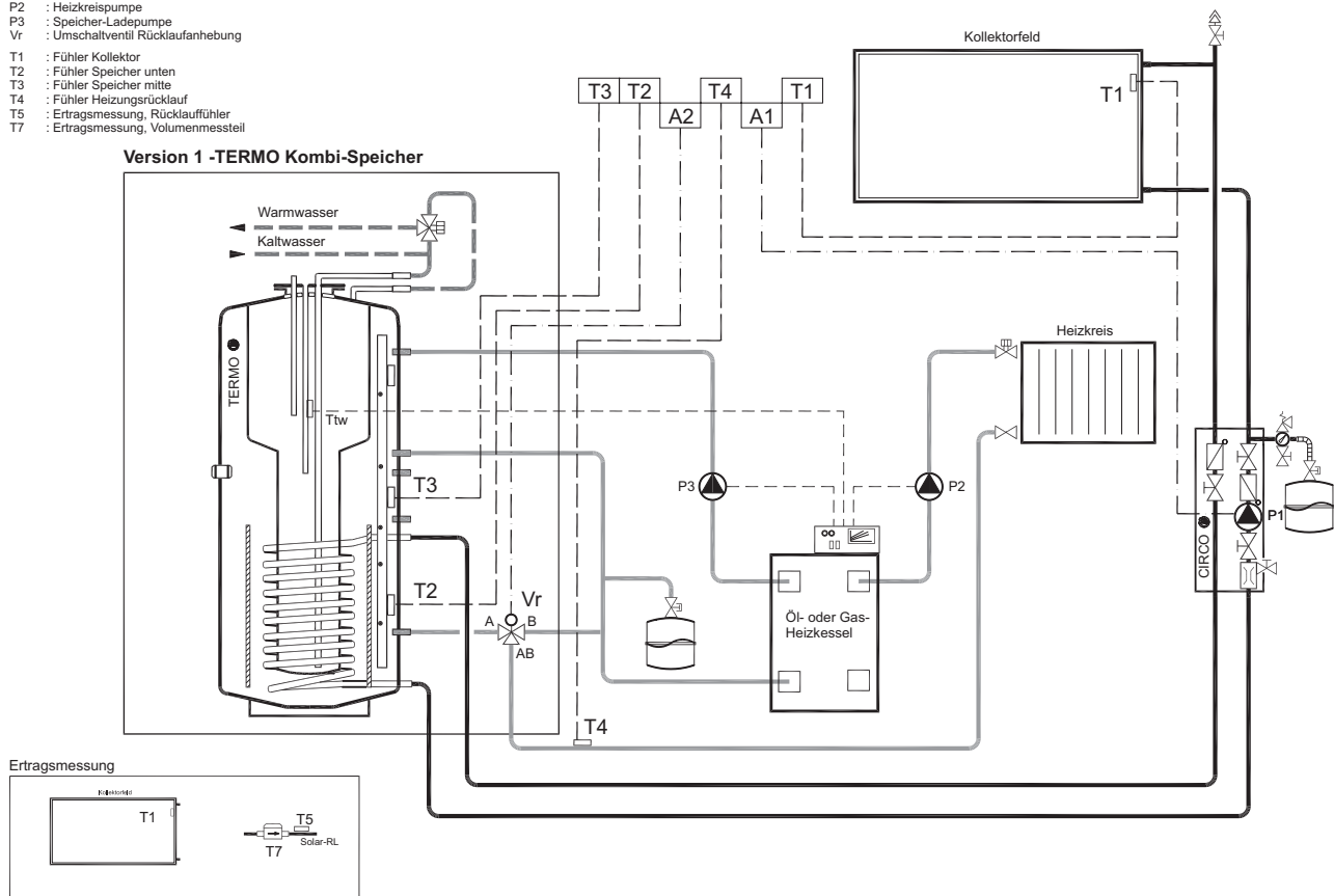
Abb. 3 Systemlösung für Warmwasserbereitung und Heizungsunterstützung. Der Regler SUNGO SL übernimmt die Speicherbeladung und die Ansteuerung des 3-Wege-Ventils für die Heizungsrücklaufanhebung.
